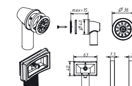
(универсальный перелив)
